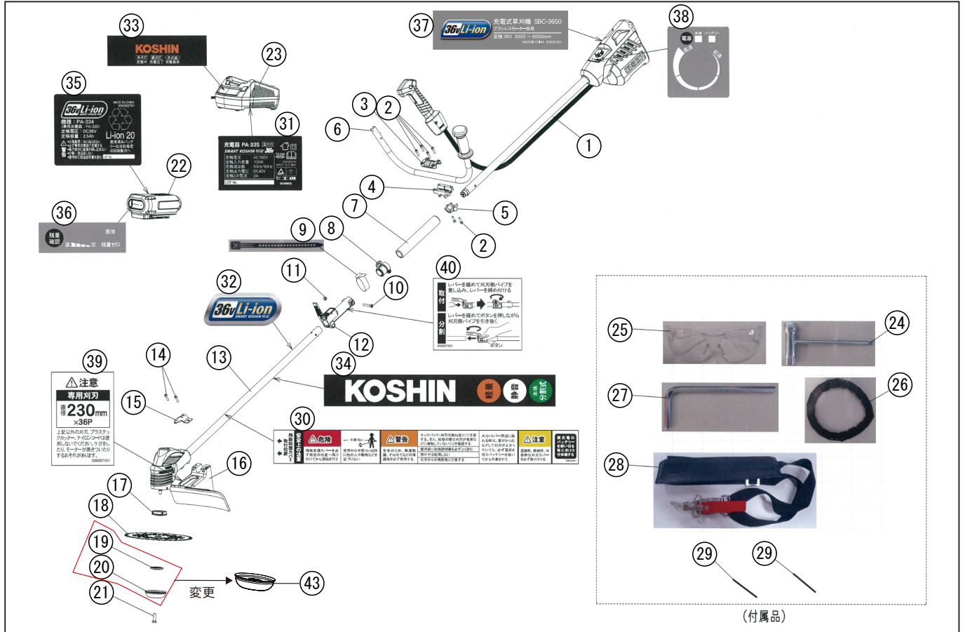
型式名 SBC-3650-AAA-0 (056855101)
